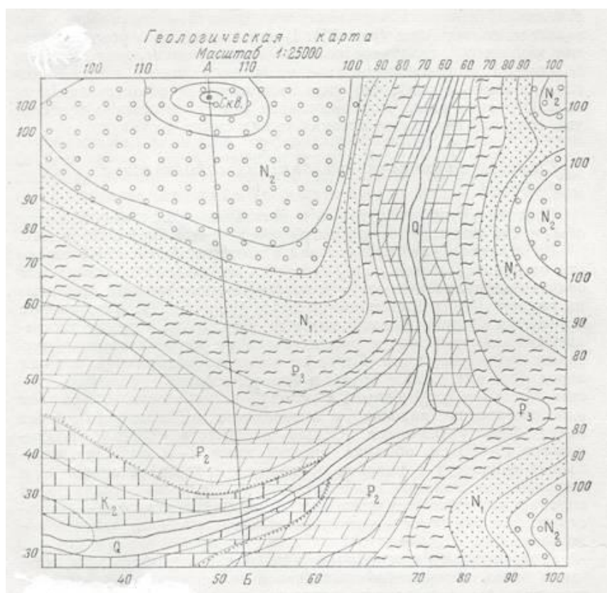
Рис. 1. Геологическая карта участка на топографической основе с горизонтальным залеганием слоев (к зад.2)
