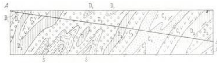
Рис. 11. Фрагмент геологической карты для района со складчатым залеганием горных пород.
