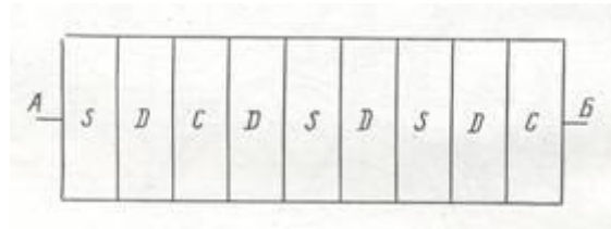
Рис. 9. Геологическая карта участка
