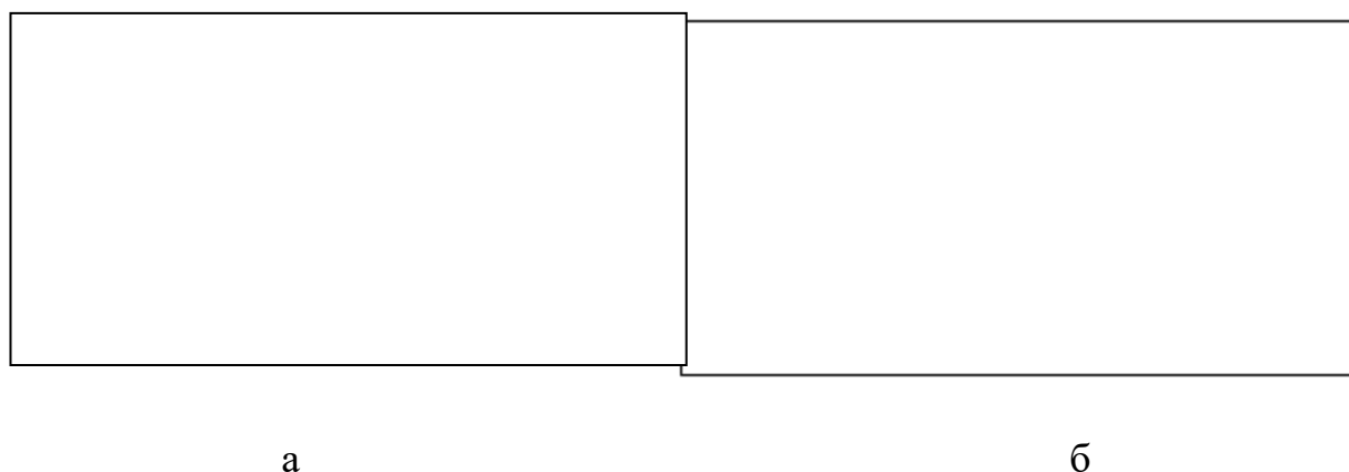
Рисунок 2 – Фотографии почвенных исследований точки №1: а – фотография точки исследования, б – почвенный профиль
