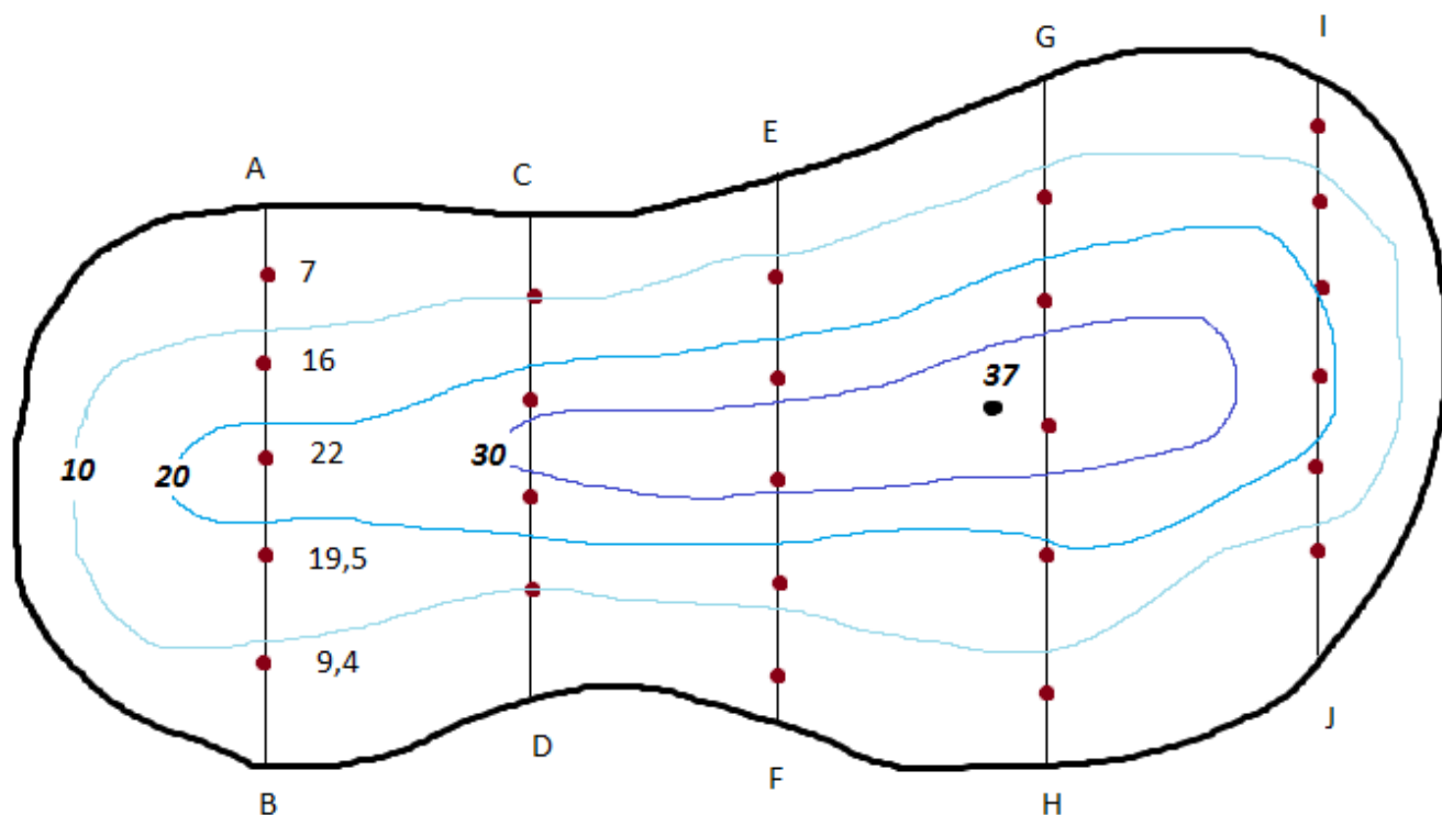
Рисунок 4 – Пример нанесения изобат озера (через каждые 10 см) по результатам полученным промером глубин методом интерполяции
