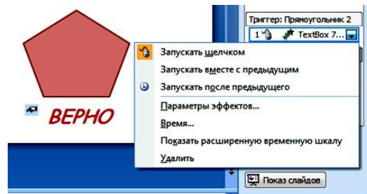
Рис. 2. Меню Textbox
