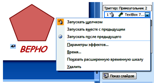
Рис.2. Меню Textbox
